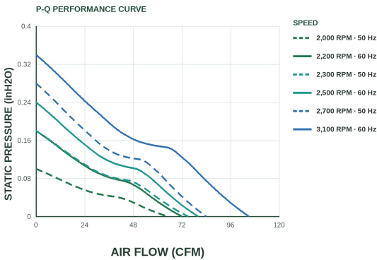
風量 - 靜壓曲線 P-Q CURVE
