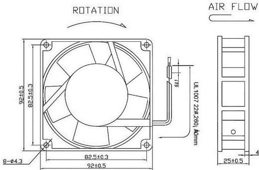
外觀尺寸圖 DIMENSIONS (mm)
