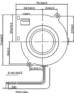
外觀尺寸圖 DIMENSIONS (mm)
