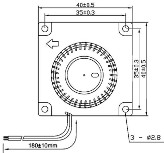
外觀尺寸圖 DIMENSIONS (mm)
