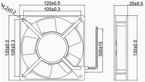
外觀尺寸圖 DIMENSIONS (mm)
