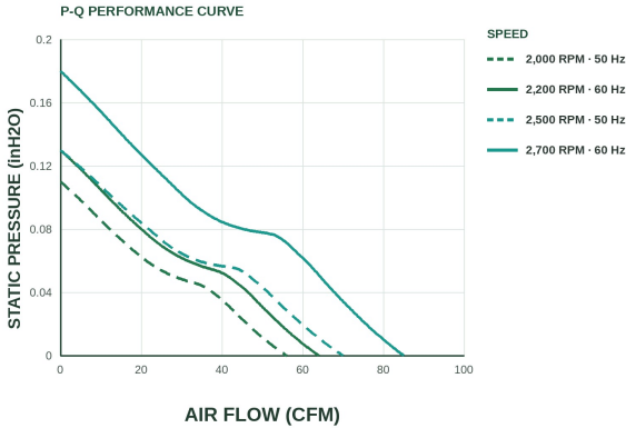
風量 - 靜壓曲線 P-Q CURVE
