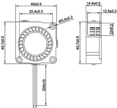
外觀尺寸圖 DIMENSIONS (mm)
