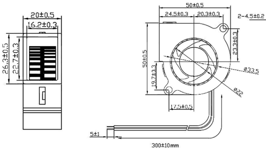
外觀尺寸圖 DIMENSIONS (mm)
