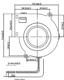
外觀尺寸圖 DIMENSIONS (mm)
