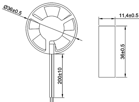
外觀尺寸圖 DIMENSIONS (mm)
