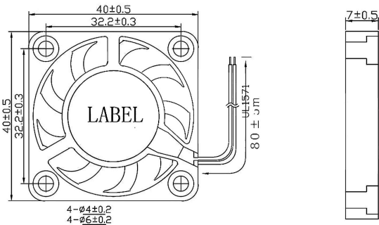
外觀尺寸圖 DIMENSIONS (mm)
