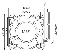
外觀尺寸圖 DIMENSIONS (mm)
