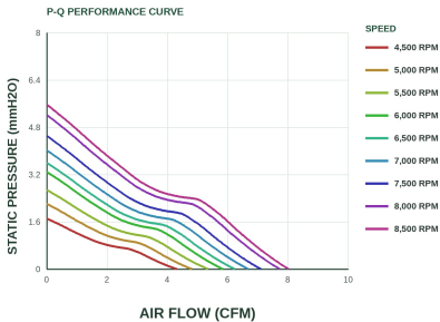
風量 - 靜壓曲線 P-Q CURVE
