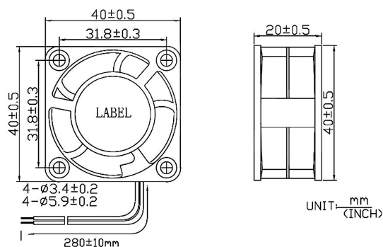
外觀尺寸圖 DIMENSIONS (mm)
