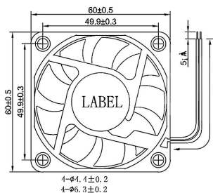
外觀尺寸圖 DIMENSIONS (mm)
