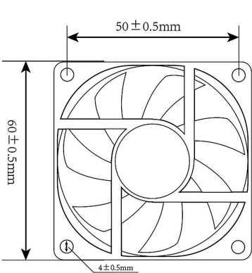
外觀尺寸圖 DIMENSIONS (mm)
