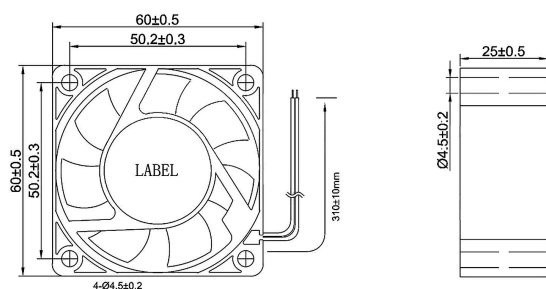
外觀尺寸圖 DIMENSIONS (mm)
