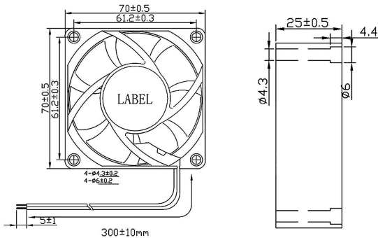
外觀尺寸圖 DIMENSIONS (mm)
