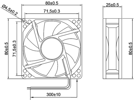
外觀尺寸圖 DIMENSIONS (mm)
