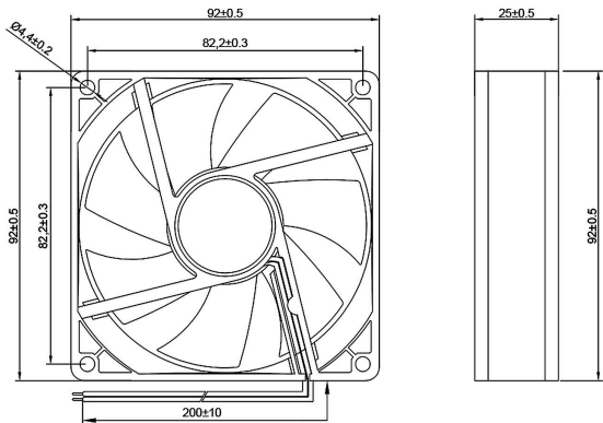
外觀尺寸圖 DIMENSIONS (mm)
