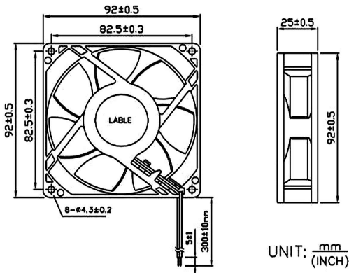
外觀尺寸圖 DIMENSIONS (mm)
