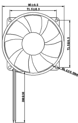
外觀尺寸圖 DIMENSIONS (mm)
