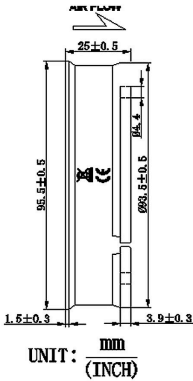
外觀尺寸圖 DIMENSIONS (mm)
