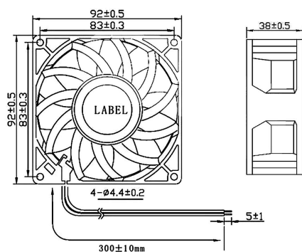
外觀尺寸圖 DIMENSIONS (mm)
