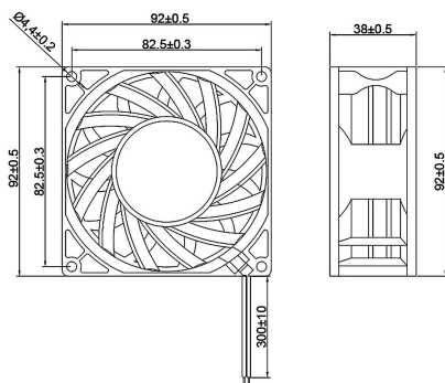
外觀尺寸圖 DIMENSIONS (mm)
